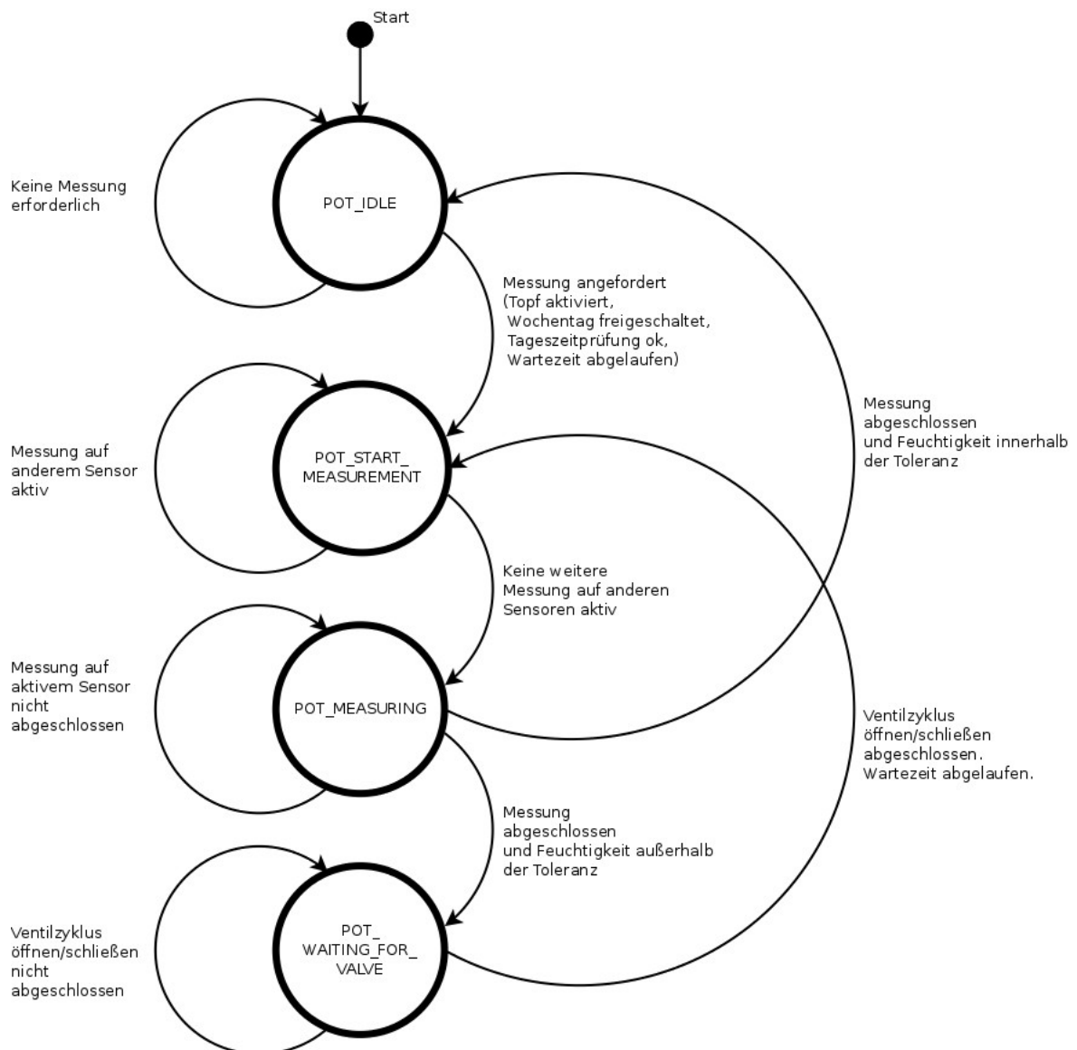
Abb. 10: Zustandsdiagramm (Regler)
